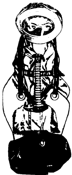
Рис. 9.3. Самоспасатель промышленный изолирующий СПИ-20
